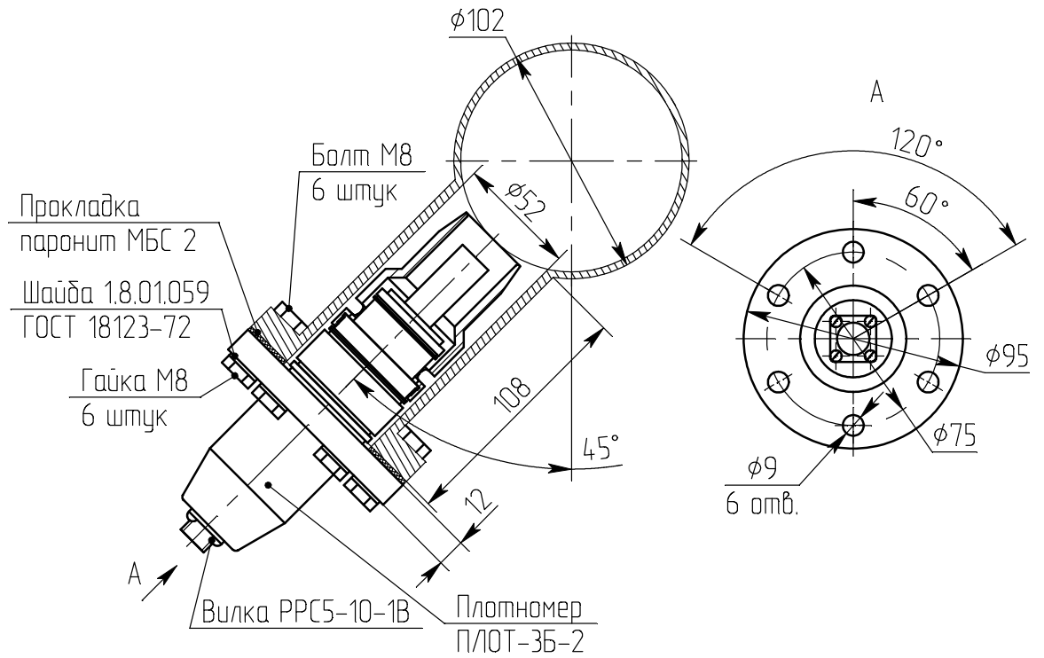
а) на горизонтальном трубопроводе
